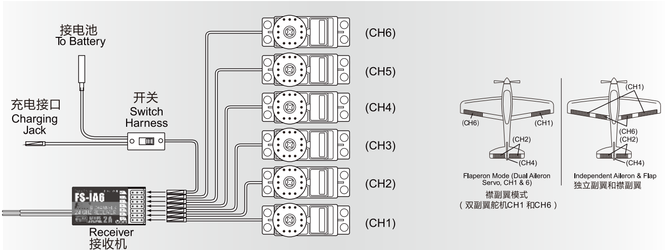
飞机模型的接收机与伺服器连接
