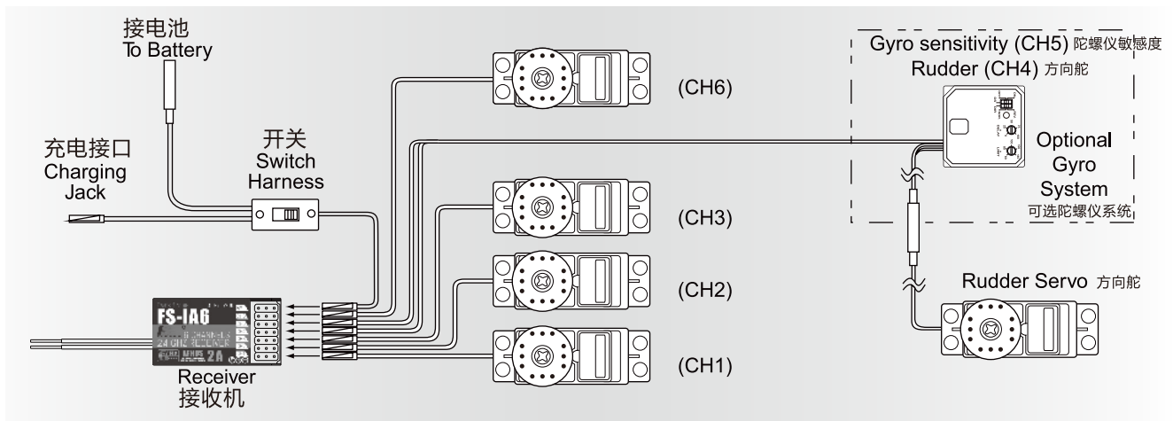
直升机模型的接收机与伺服器连接
