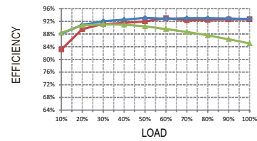
RSD-60L-5
